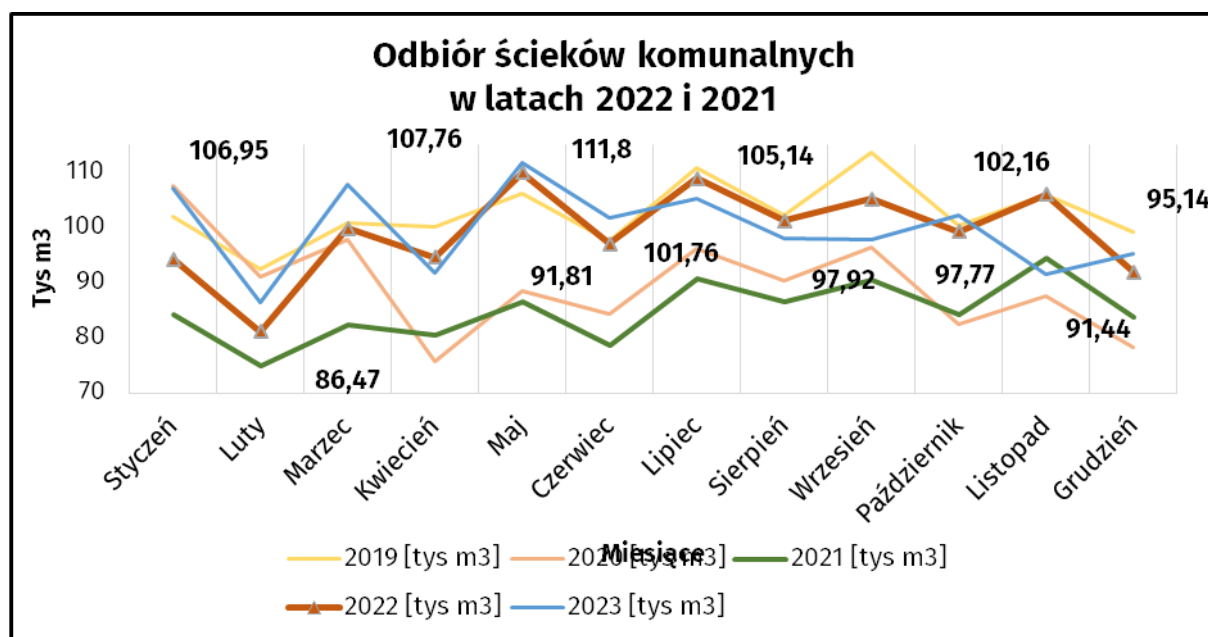
Wyk. Ilość odprowadzonych ścieków w roku 2023, w porównaniu do lat 2019-2022
